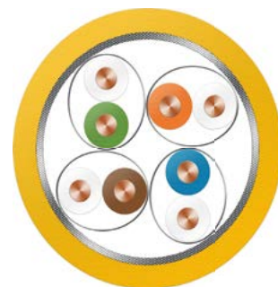
MegaLine® S/FTP Querschnittszeichnung simplex
