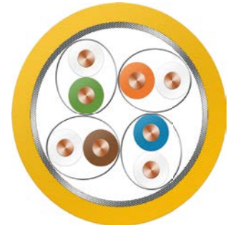
MegaLine® S/FTP Querschnittszeichnung simplex
