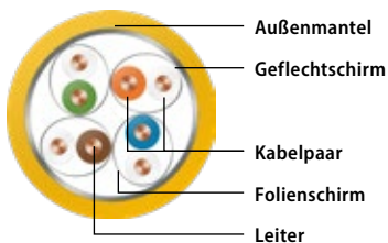
S/FTP (PiMF mit Gesamtschirm)
